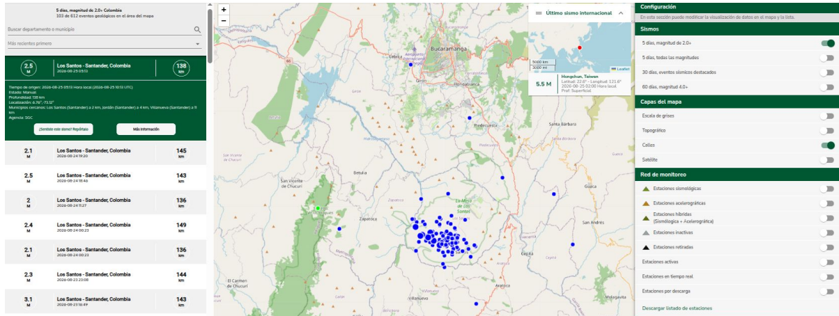
Figura 1. Visor de sismos del Servicio Geológico Colombiano.
