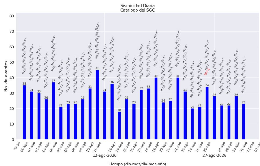
Figura 2. Sismicidad diaria de agosto, en un radio de 30 km alrededor de Los Santos, Santander.
