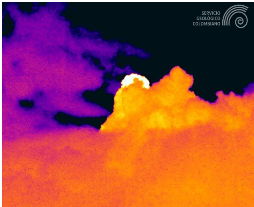
Figura 1. Registro de la cámara Mina IR, ubicada a 2,2 km en dirección norte del volcán Puracé que muestra una emisión de gases registrada el 2 de enero a las 1:16 a. m. (hora local).
