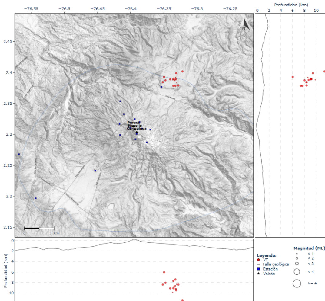
Figura 1. Mapa de localización de eventos sísmicos tipo VT registrados entre las 2:00 p. m. del 13 de septiembre y las 2:00 p. m. del 14 de septiembre de 2026.
