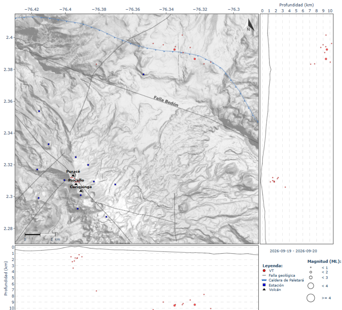
Figura 1. Mapa de localización de eventos sísmicos tipo VT registrados entre las 2:00 p. m. del 19 de septiembre y las 2:00 p. m. del 20 de septiembre de 2026.
