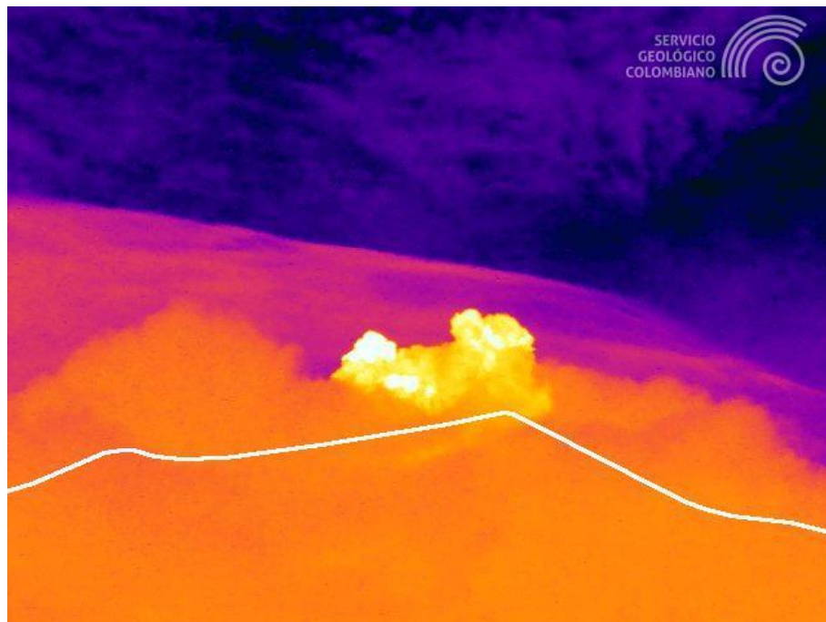
Figura 2. Registro de la cámara térmica Mina2IR ubicada 2,2 km al norte del volcán Puracé, que muestra el contorno del volcán Puracé delineado de color blanco, y una emisión de ceniza registrada el 5 de septiembre de 2026 a las 8:00 p. m.
