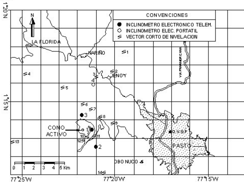
Figura 2.18. Red de vigilancia en Deformación del Volcán Galeras. Inclínómetros electrónicos: 1: Cráter, 2: Peladitos, 3: Huairatola, 4: Chorrillo (portátil). Vectores cortos de nivelación: 1: Puyito, 2: Lindero, 3: Chorrillo, 4: Chacaguaico, 5: Barranco, 6: Chiguaco, 7: Popeye, 8: Piedras, 9: La Mica, 10: La Y, 11: Inclínómetro, 12: Telecom, 13: La Quebrada, 14: Cobanegra.
