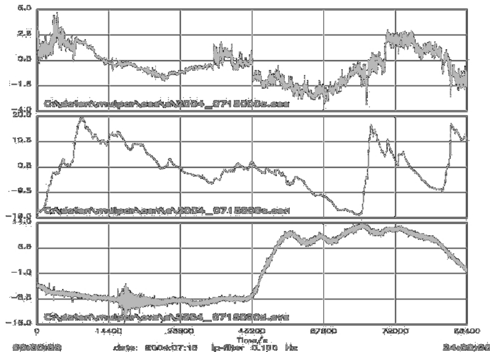
Figura 2.56 Comportamiento regular de las componentes horizontales del campo eléctrico (superior) CEE, (medio) CEN y registro sísmológico de la componente vertical de la estación ANGANÓY, correspondiente al día 15 de julio de 2004. Las gráficas muestran valores relativos de amplitud en unidades reales de \mu\text{V} \times \text{m} , en el campo eléctrico.
