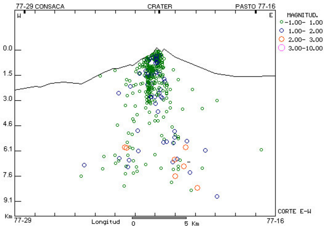
Figura 2.10. Distribución hipocentral de sismos VT, corte oeste-este. Julio a diciembre de 2004.
