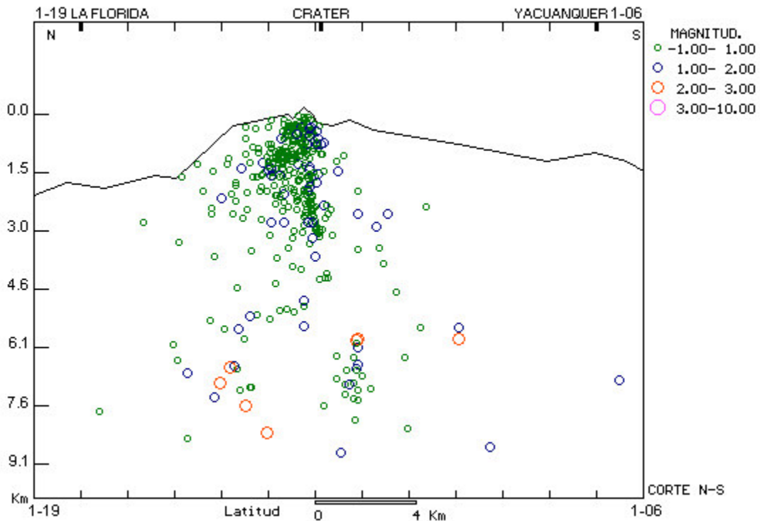
Figura 2.11. Distribución hipocentral de sismos VT, corte norte-sur. Julio a diciembre de 2004.
