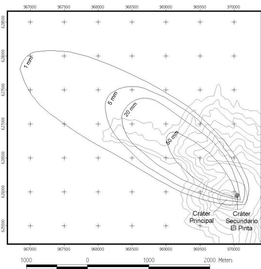
Figura 2.72 Distribución de caída piroclástica. Emisión de cenizas de julio 21
