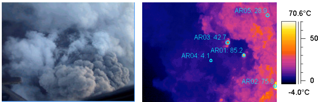
Figura 2.79 Fotografías digital y térmica tomadas en el cono activo de Galeras en septiembre 7 de 2004
