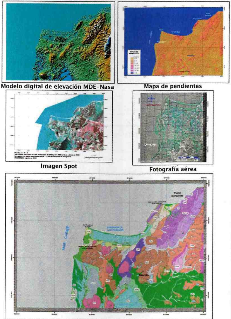
Figura 5. Información temática básica tenida en cuenta en la elaboración de la plancha geomorfológica 16-IV-D escala 1:25.000. Nótese la diferenciación de unidades de origen marino en tonos de verde, origen morfoestructural en púrpuras, origen denudacional en marrón.
