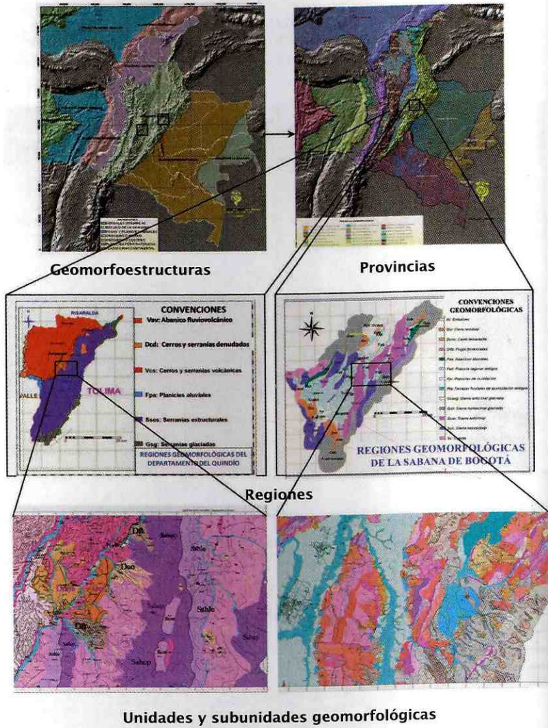
Figura 3. Ejemplo de la visión taxonómica geomorfológica propuesta, con aplicación en Colombia.
