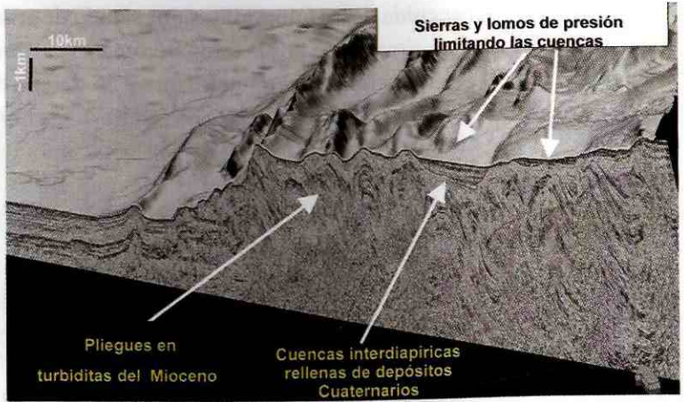
Figura 6. Ejemplo de la información obtenida de la combinación de imágenes de sonar de barrido lateral (ecosonda multihaz y perfiles sísmicos de reflexión al SW de Cartagena).
