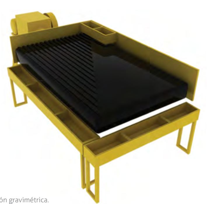
Fotografía 11: Modelo de mesa de concentración. Fuente: Propia.
