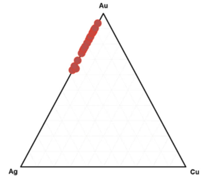
Figura 4.21: Diagrama triangular Au-Ag-Cu, para las partículas de oro analizadas con microsonda electrónica, La Llanada. Fuente: Propia.
