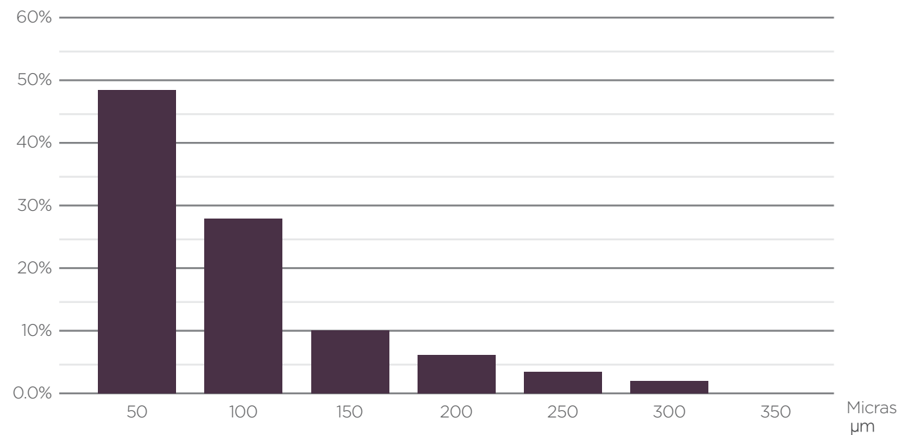
Figura 4.20: Distribución de oro en peso por rangos de tamaño zona de la Llanada. Fuente: Propia.
