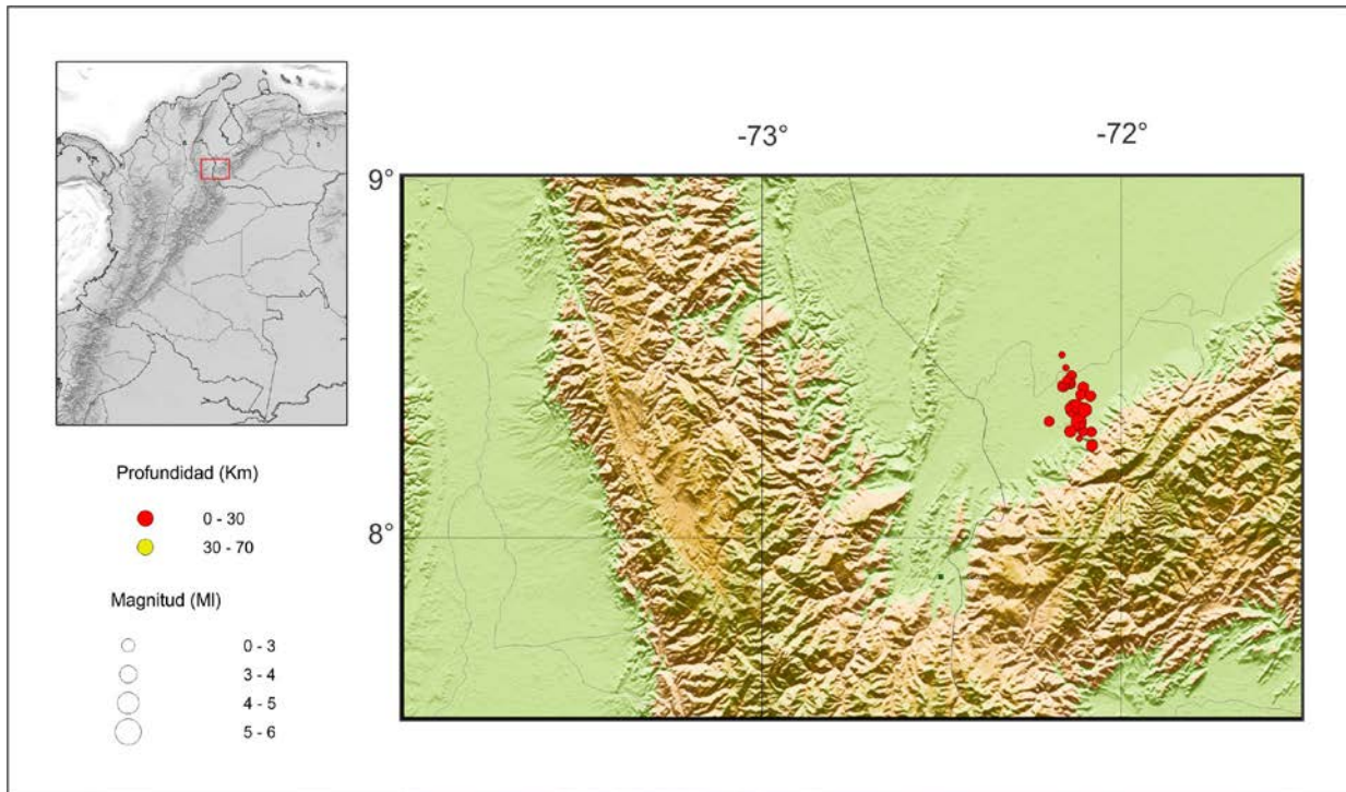
Figura 1. Mapa de réplicas con MI > 3.0 del sismo del 05 de Febrero de 2015 en la Frontera Colombia-Venezuela
