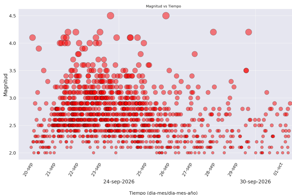
Figura 6. Distribución de la magnitud de los sismos registrados en Chaparral, Tolima, en función del tiempo, desde el 20 de septiembre de 2026. Cada círculo representa un sismo y su tamaño es proporcional a la magnitud.
