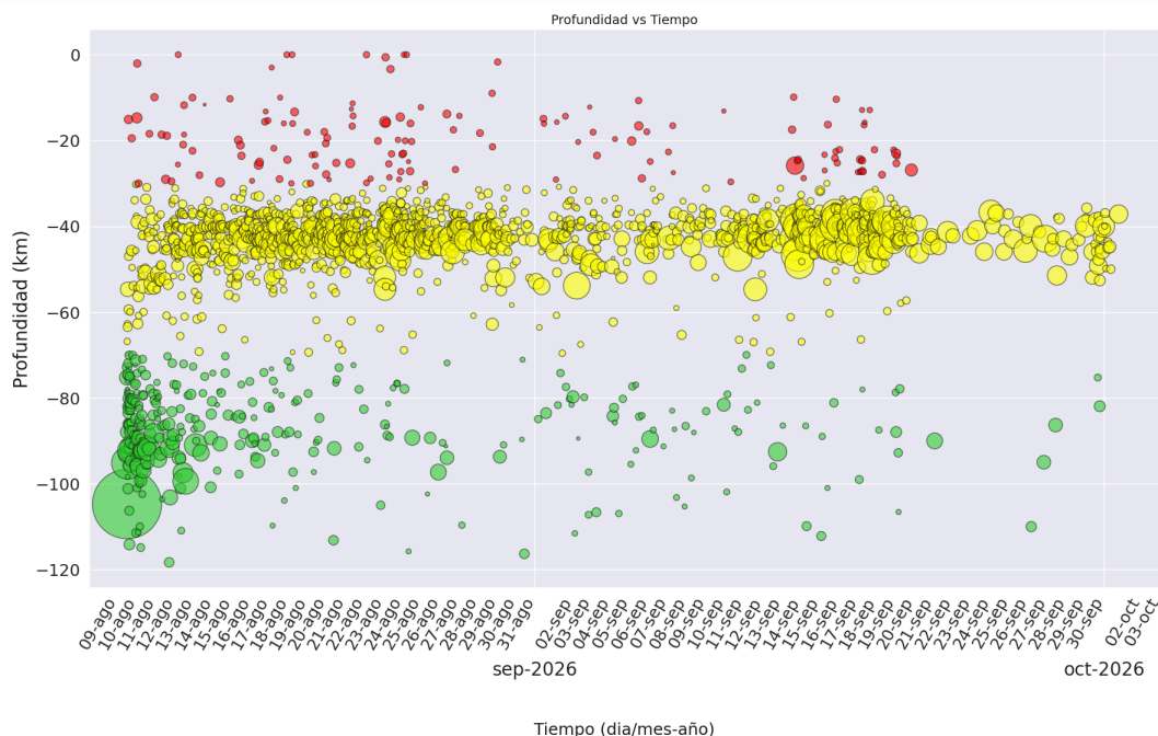
Figura 2. Evolución en el tiempo y en profundidad de la sismicidad registrada desde el 10 de agosto de 2026. Cada círculo representa un sismo; su tamaño es proporcional a la magnitud y los colores indican diferentes rangos de profundidad.
