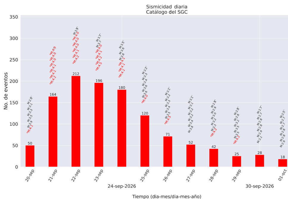
Figura 5. Número diario de sismos de magnitud mayor a 2,0 registrados en Chaparral, Tolima, desde el 20 de septiembre de 2026. Sobre cada barra se indica el total de eventos diarios y, en la parte superior, las magnitudes de los sismos más destacados de cada día; en rojo se resaltan los eventos de magnitud igual o superior a 4,0. La información del 30 de septiembre corresponde al corte de las 5:00 p. m.
