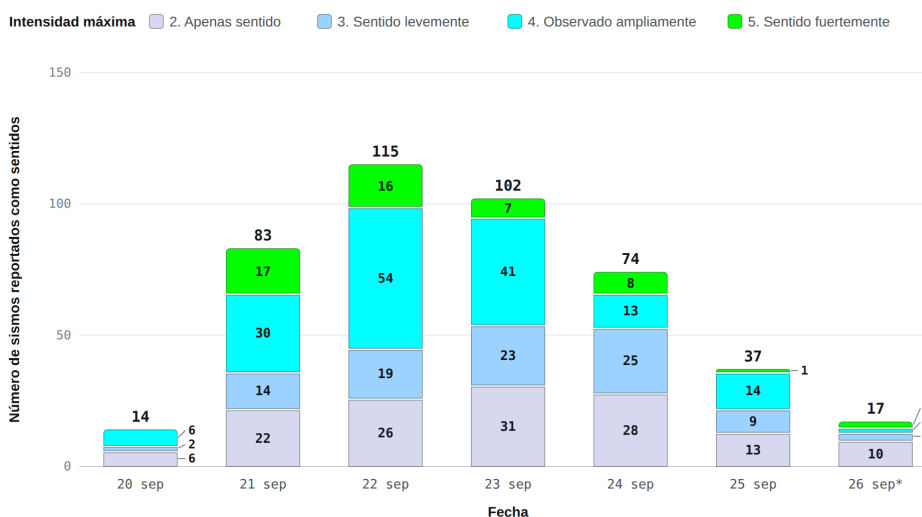
Número de sismos sentidos diarios según su intensidad
