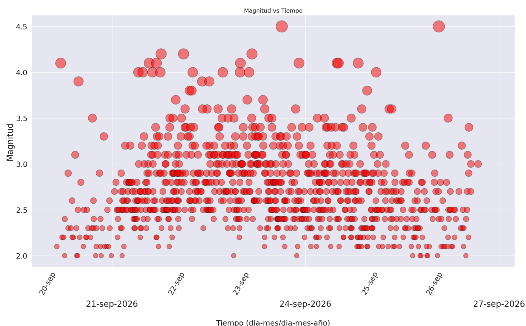
Figura 6. Distribución de la magnitud de los sismos registrados en Chaparral, Tolima, en función del tiempo, desde el 20 de septiembre de 2026. Cada círculo representa un sismo y su tamaño es proporcional a la magnitud.
