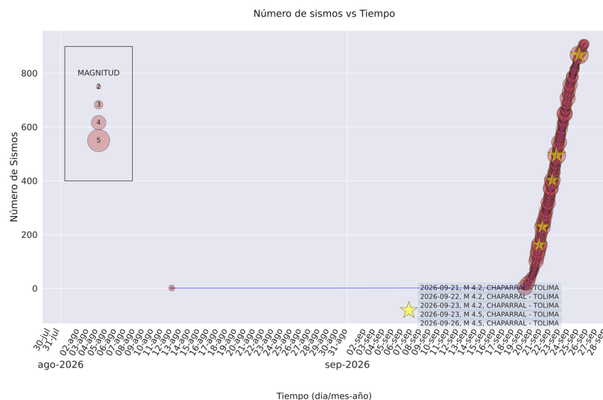
Figura 4. Evolución del número de sismos registrados en Chaparral, Tolima desde agosto de 2026. Cada círculo representa un sismo; su tamaño es proporcional a la magnitud; las estrellas representan los sismos de mayor magnitud.
