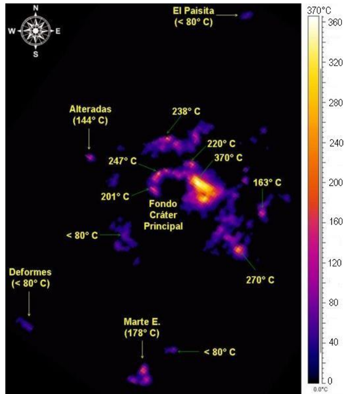
Figura 2.60. Imagen Térmica, septiembre 27 de 2007, 06:15 a.m.
