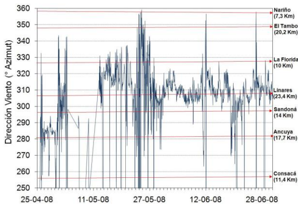
Figura 2.66. Comportamiento de los valores de dirección del viento en la cima de Galeras. Abril a junio de 2008.
