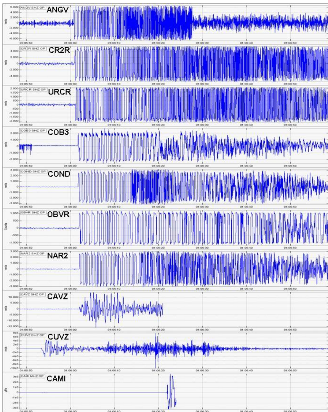
Figura 2.10. Registro sísmico de la erupción de enero 17 de 2008, a las 8:06 p.m. en las estaciones de corto periodo Anganoy, Cráter-2, Urcunina, Cobanegra, Cónдор, Obonuco, Nariño y Calabozo, en la estación de banda ancha Cufiño y registro acústico en la estación CAMI.
