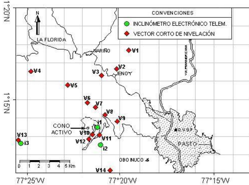
Figura 2.20. Red de vigilancia en Deformación del Volcán Galeras. Inclinómetros electrónicos: i1: Cráter, i2: Peladitos, i3: Calabozo. Vectores cortos de nivelación: V1: Puyito, V2: Lindero, V3: Chorrillo, V4: Chacaguaico, V5: Barranco, V6: Chiguaco, V7: Popeye, V8: Piedras, V9: La Mica, V10: La Y, V11: Inclinómetro, V12: Telecom, V13: La Quebrada, V14: Cobanegra.
