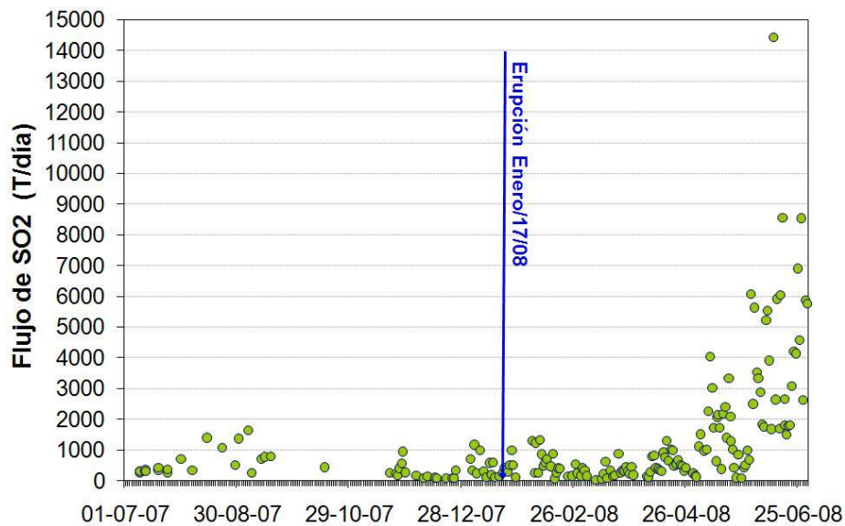
Figura 2.37. Flujo de SO 2 de Galeras, medido con estaciones Scan-DOAS (NOVAC). Junio de 2007 a julio de 2008.
