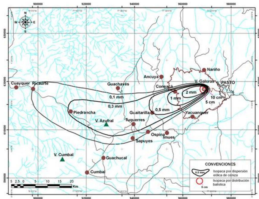
Figura 2.17. Mapa de distribución eólica de las cenizas producidas en la erupción de enero 17 de 2008, de acuerdo con las inspecciones en campo por personal de INGEOMINAS. Las isópacas de dispersión eólica están en mm y las de dispersión balística en cm.
