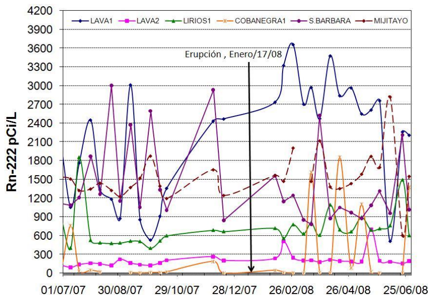
Figura 2.40. Emisiones de Rn-222, en la Línea Galeras. Julio de 2007 a junio de 2008.
