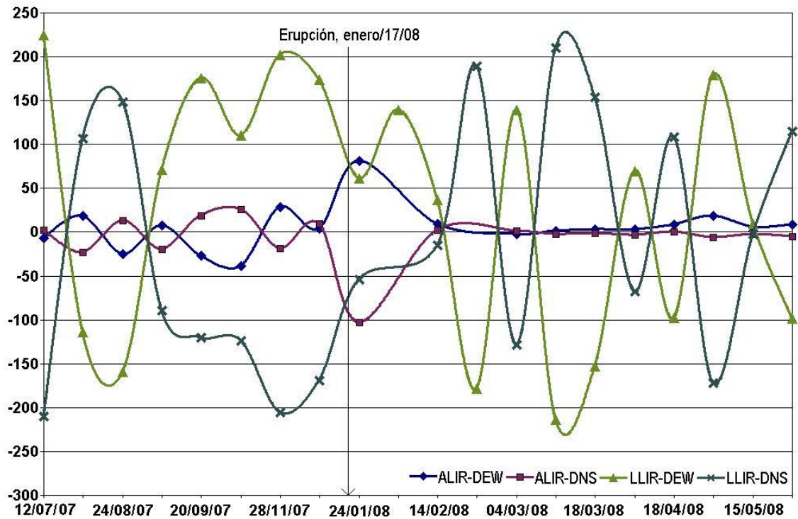
Figura 2.42. PEE medido en las componentes horizontales de la estación Lirios. Julio de 2007 a junio de 2008.
