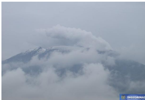
Figura 2.54. Emisión de gases, se observa granizo en la cima por las bajas temperaturas. 13/Mar/11:47 a.m.
