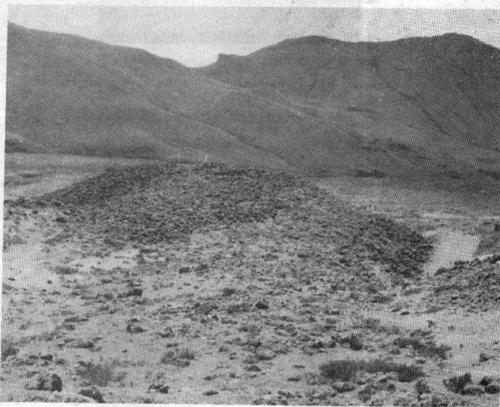
Figura 6: Flujo piroclástico más reciente del volcán Puracé (1869?). Sector NW, quebradas Agua Blanca, Chagartón.
