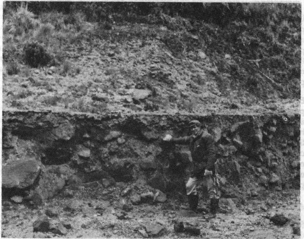
Figura 8: Cenizas de caída y bombas de las últimas erupciones. Sector: Parte alta río Anambío.
