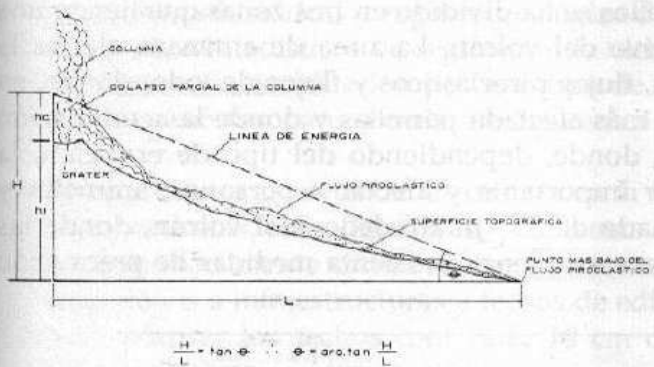
Figura 12: Esquema que ilustra el concepto de la línea de energía.
