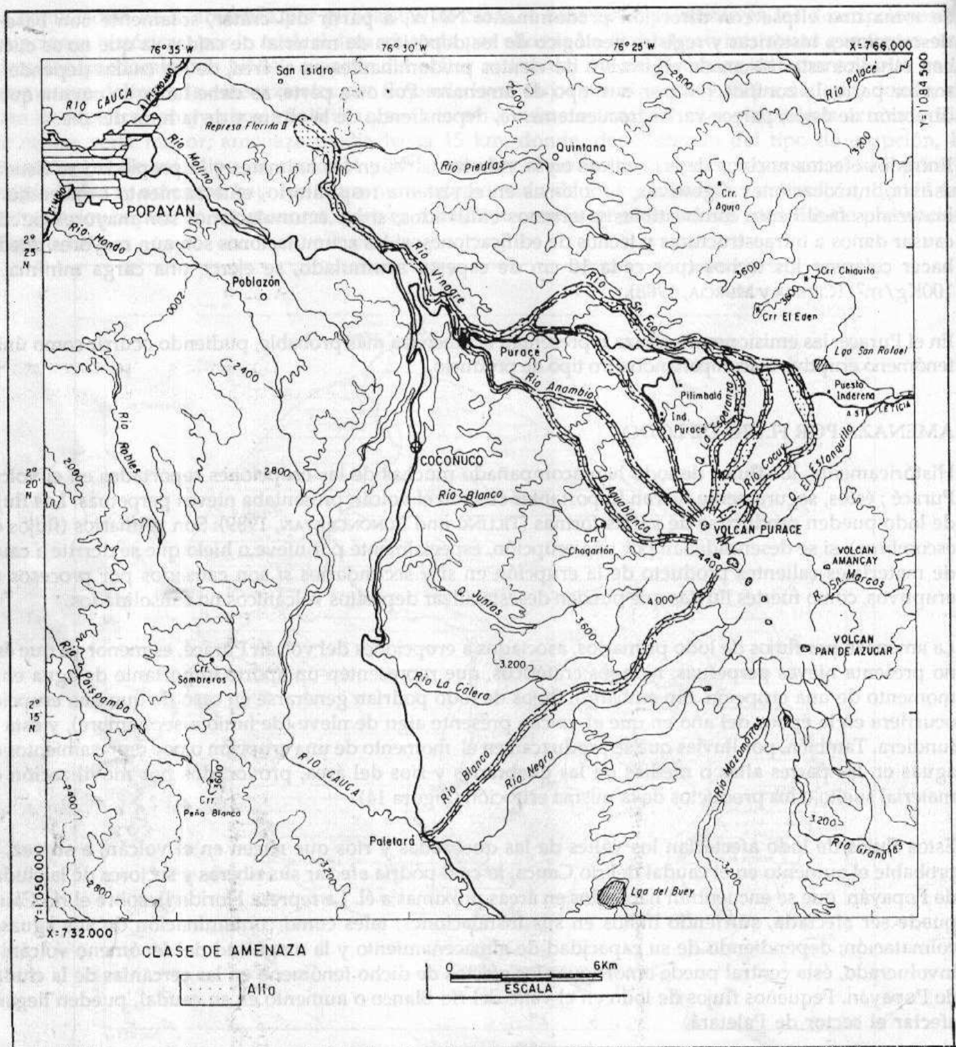
Figura 14: Mapa de amenaza por flujos de lodo del volcán Puracé.
