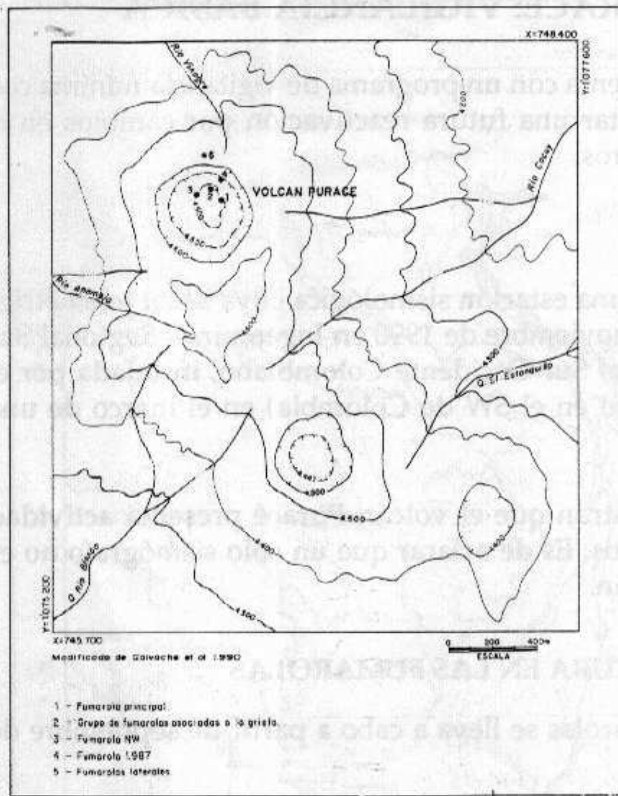
Figura 16: Localización de las fumarolas asociadas al volcán Puracé.
