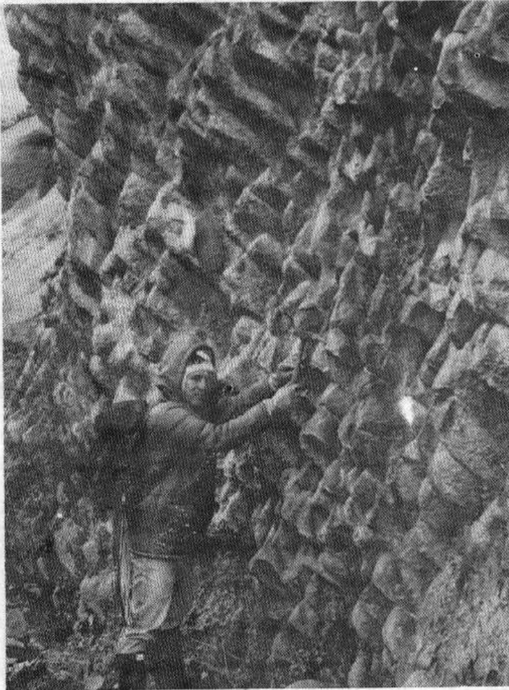
Figura 4: Coladas de lava andesítica con disyunción columnar perteneciente al estadio Puracé actual. Sitio: "El Espinazo". Flanco norte.
