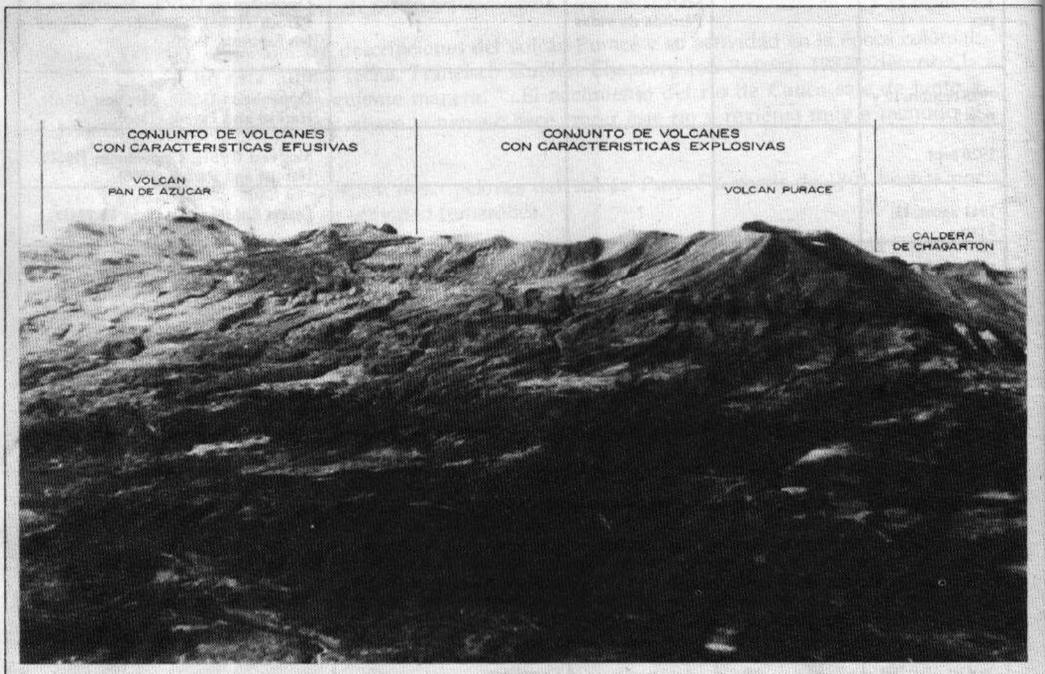
Figura 2: Cadena volcánica de Los Coconucos (Foto: Guillermo Cajiao).
