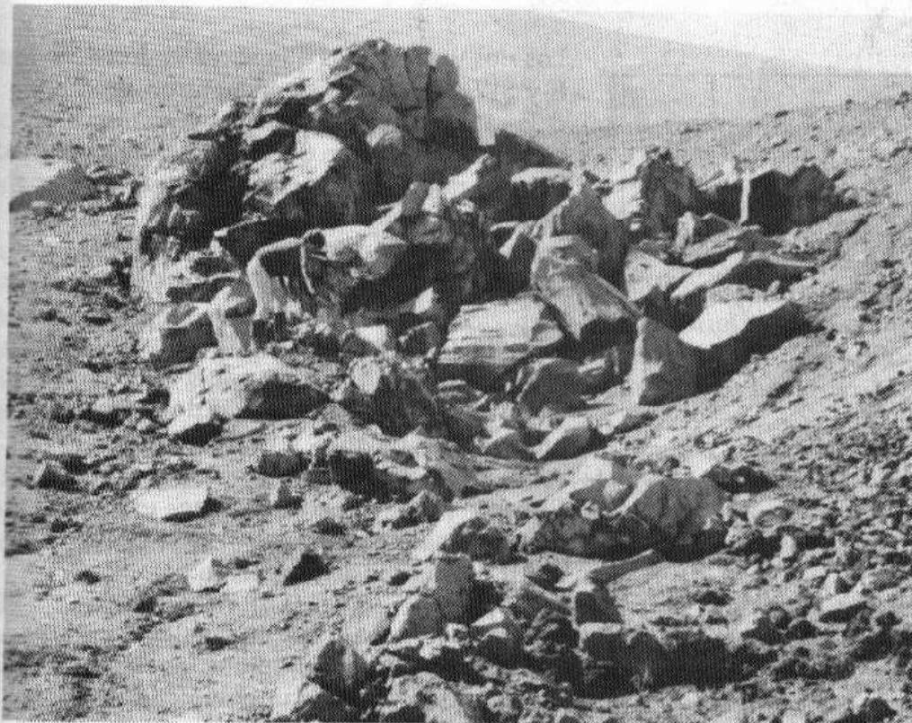
Figura 9: Posible flujo de lodo (?) o flujo de escombros asociado al volcán Puracé. Sector: Parte alta río Anambío.
