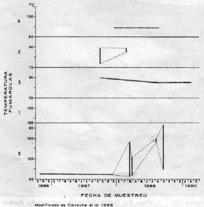
Figura 17: Temperatura de fumarolas en el volcán Puracé.
