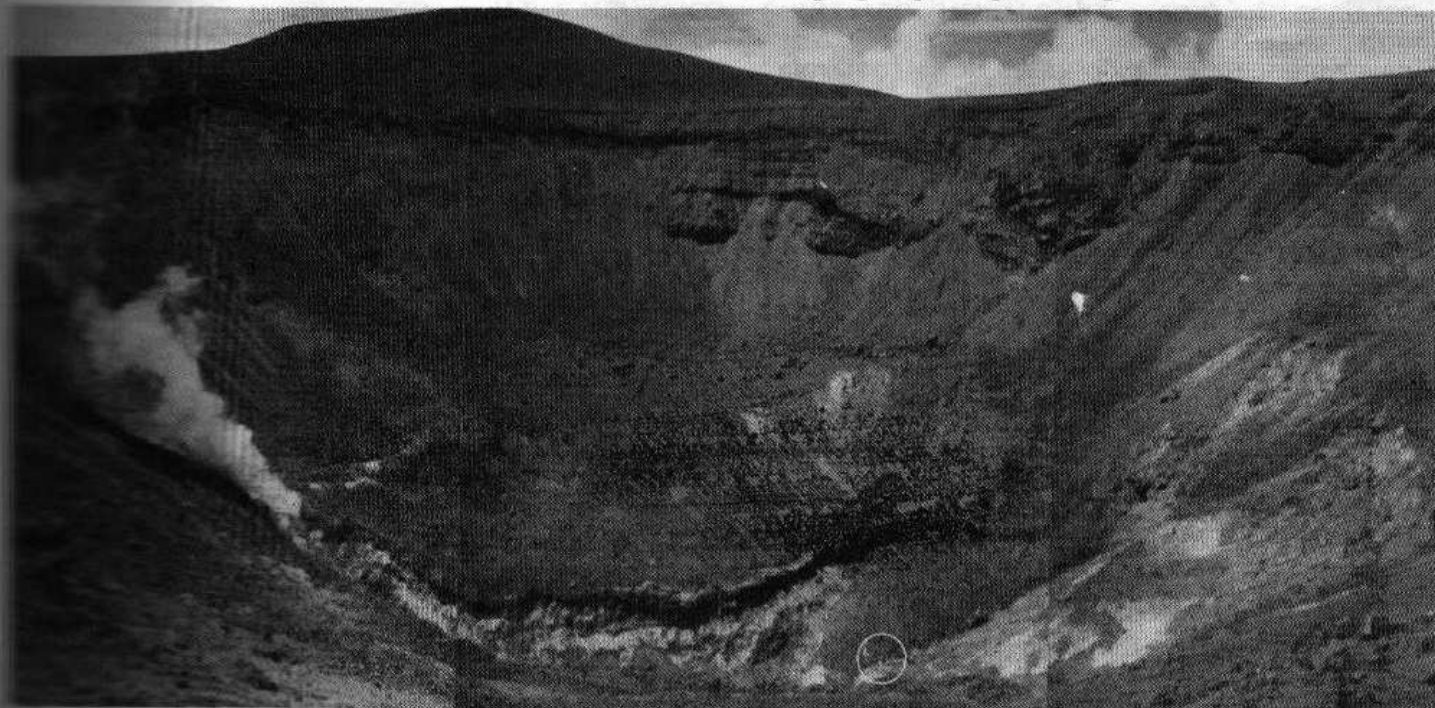
Figura 15. Vista del fondo del cráter del volcán Puracé (septiembre, 1987). En primer plano la grieta y la fumarola principal. Las personas en el círculo dan la escala aproximada. En segundo plano dos pequeños cráteres de explosión. Al fondo de la foto, borde del cráter externo del Puracé actual.
