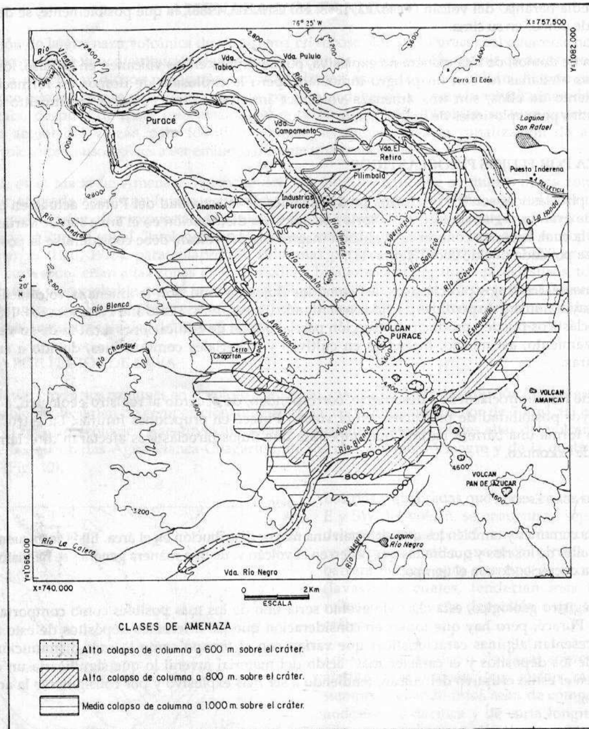
Figura 11: Mapa de amenaza por flujos piroclásticos del volcán Puracé.
