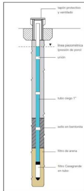
Figura 6. Esquema del piezómetro tipo Casagrande (Fuente: SISGEO, 2016)
