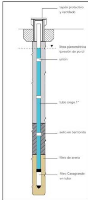
Figura 6. Esquema del piezómetro tipo Casagrande (Fuente: SISGEO, 2016)
