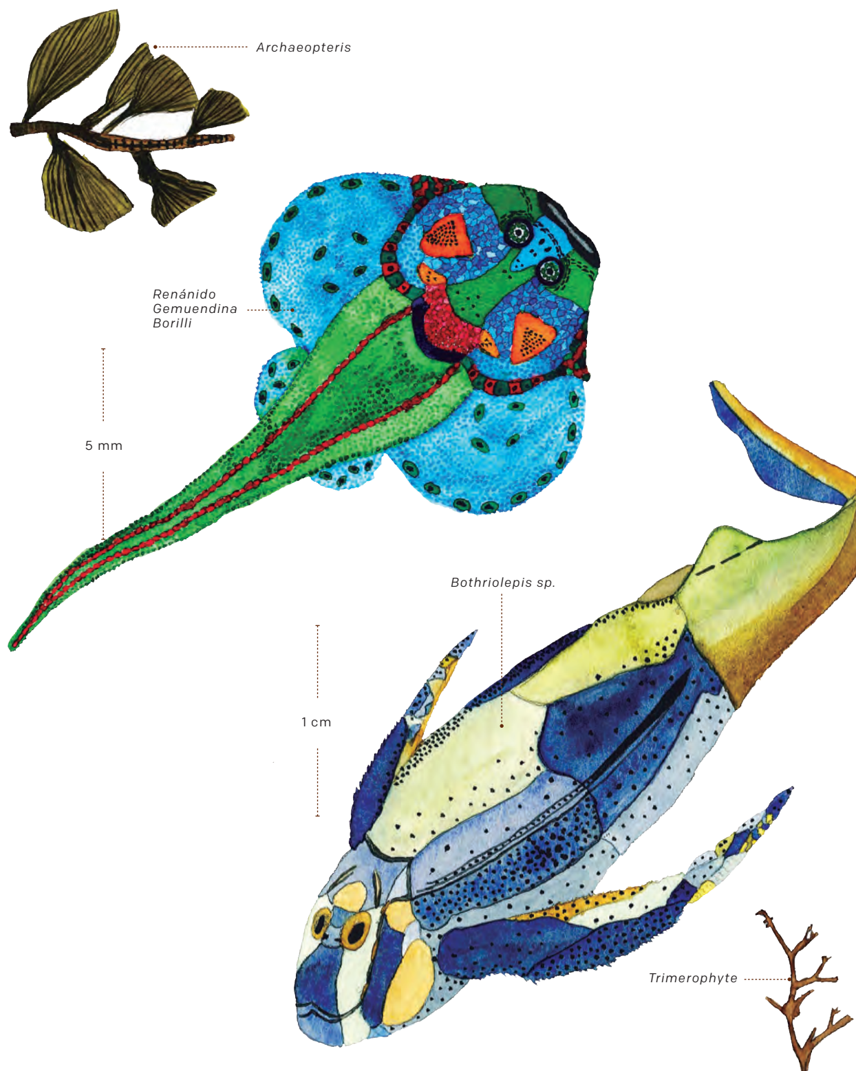
✚ Fósiles de peces marinos de la Formación Floresta y plantas de la Formación Cuche. Pintura de Karina Andrea Portilla Mendoza
