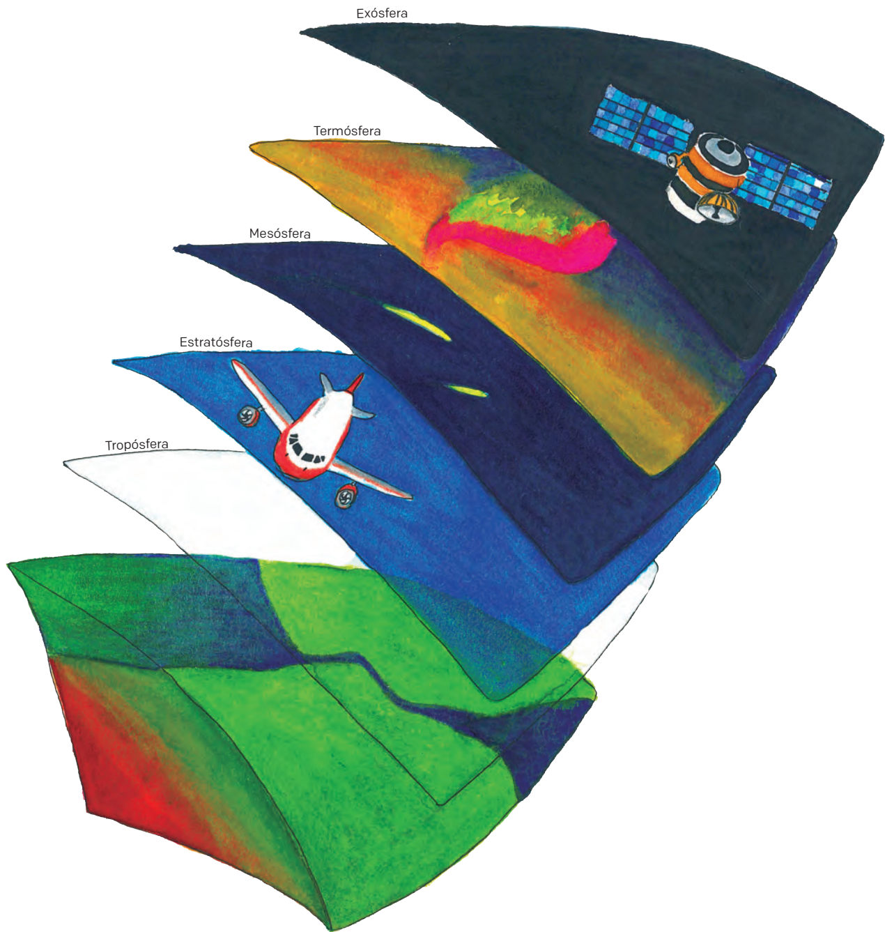
+ Esquema de la atmósfera en el sistema Tierra. Pintura de Karina Andrea Portilla Mendoza
