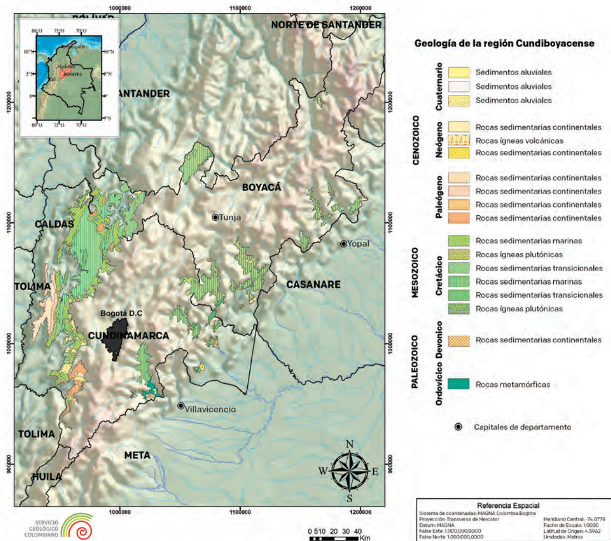
Geología de la región cafetera Cundiboyacense. Adaptado por Catalina Sánchez Caballero del Mapa Geológico de Colombia 2015, escala 1:1000000, Servicio Geológico Colombiano
